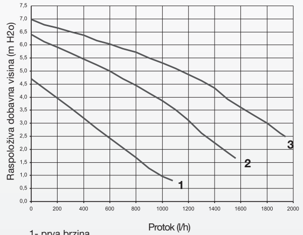
RASPOLOŽIVA DOBAVNA VISINA U KRUGU NISKE TEMPERATURE
