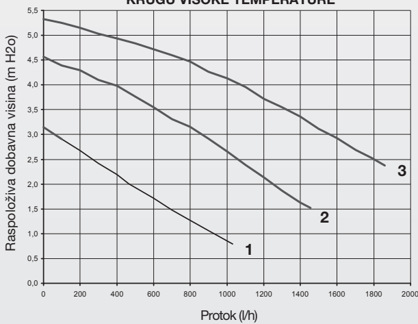
RASPOLOŽIVA DOBAVNA VISINA U KRUGU VISOKE TEMPERATURE
