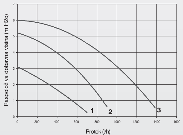
RASPOLOŽIVA DOBAVNA VISINA U KRUGU NISKE TEMPERATURE
